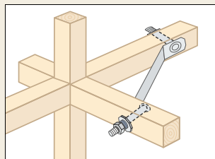
火打ち金物
