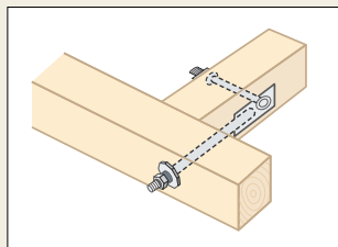
羽子板ボルト
