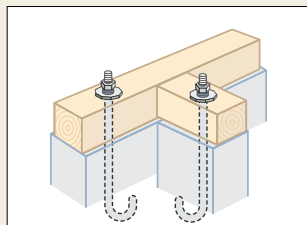
アンカーボルト
