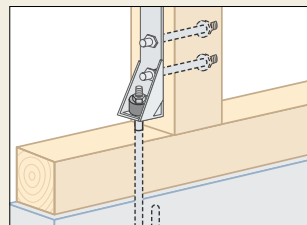
ホールダウン金物
